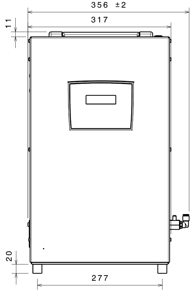
Front View Scale: 1:5
