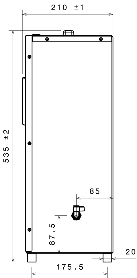
Right view Scale: 1:5
